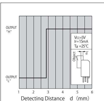
検出位置特性1(代表例) KI3193
