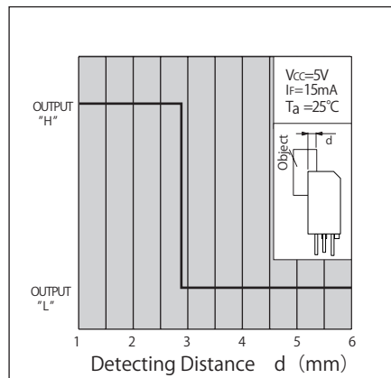
検出位置特性2(代表例) KI3193
